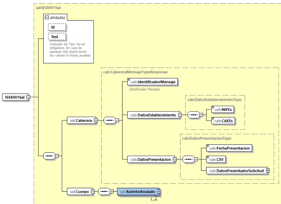
Figura 5: Bloque Anulación
