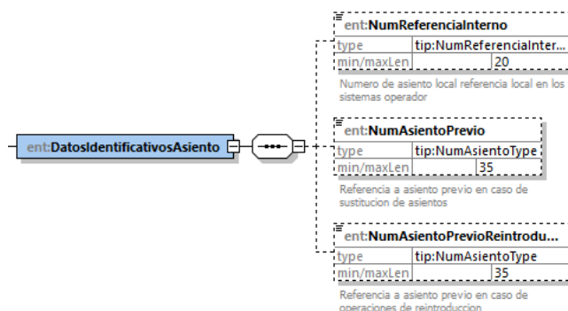
Figura 5: Datos Identificativos del Asiento
