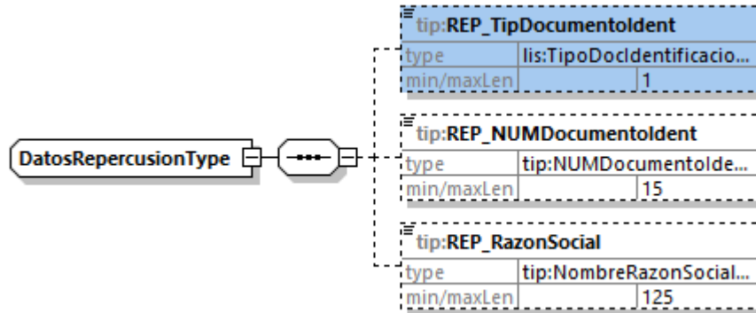
Figura 10: Datos de Repercusión
