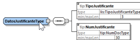
Figura 8: Datos del Documento
