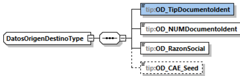
Figura 9: Datos Origen/Destino
