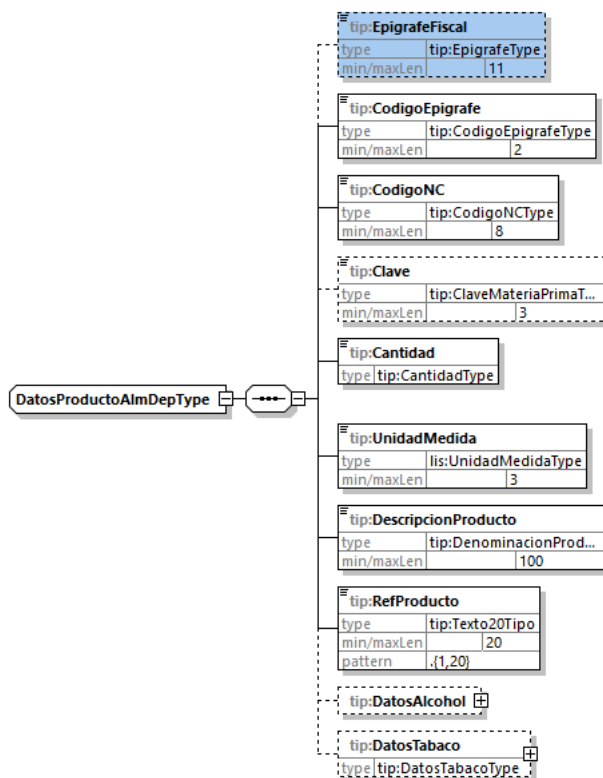
Figura 11: Datos del Producto
