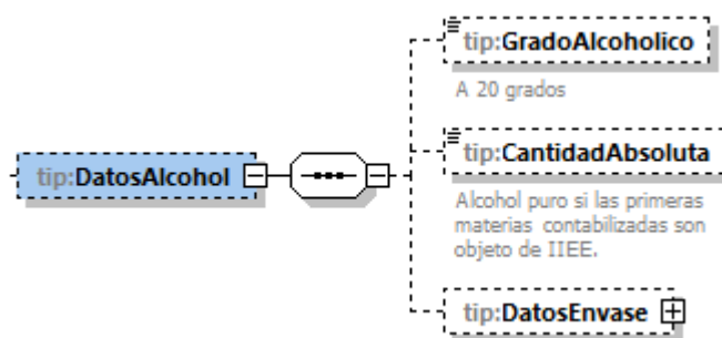
Figura 12: Bloque Datos Alcohol
