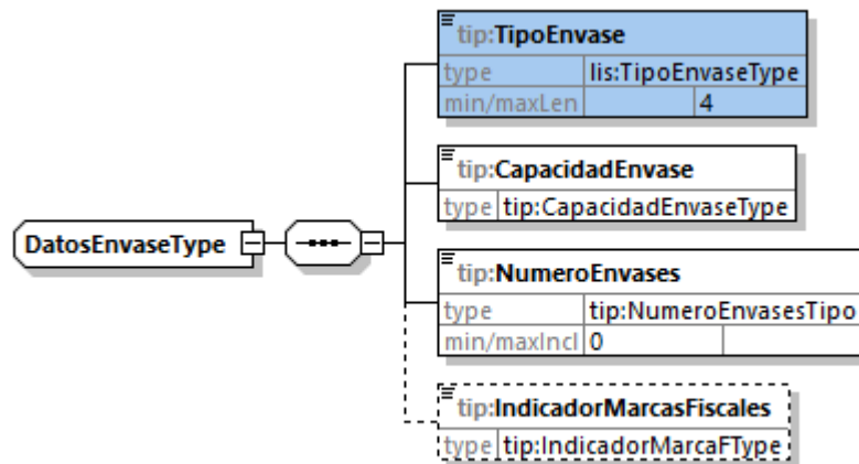
Figura 13: Datos del Envase
