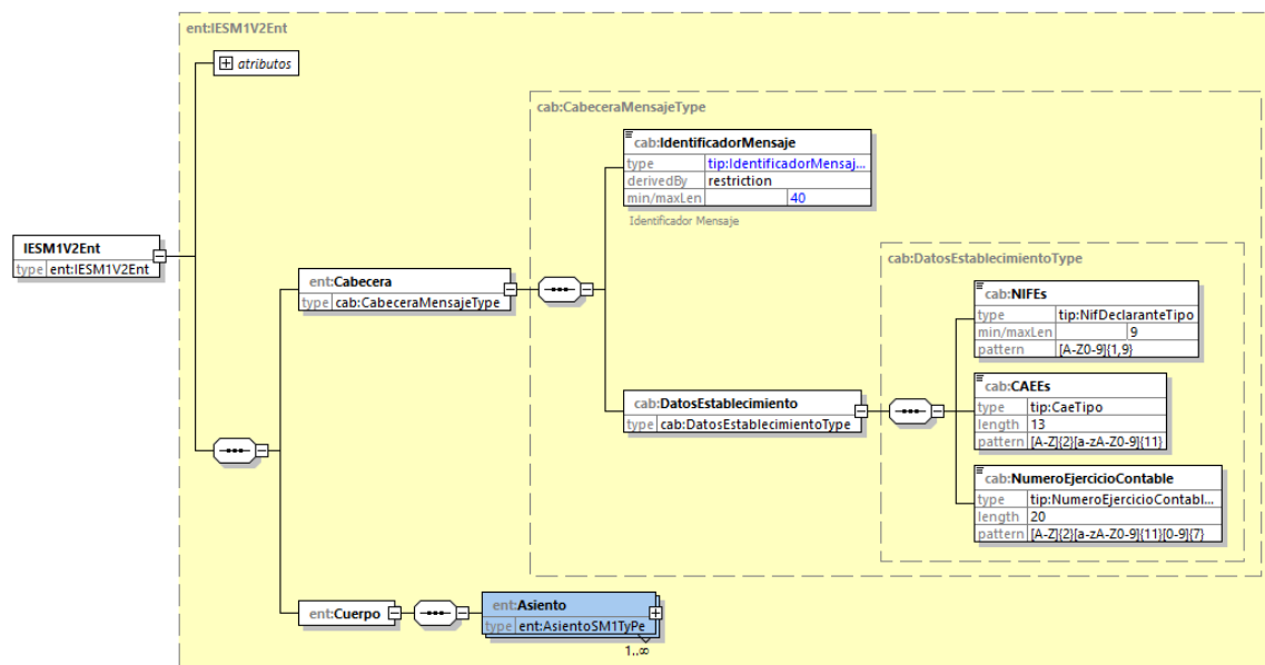
Figura 3: Mensaje de Entrada
