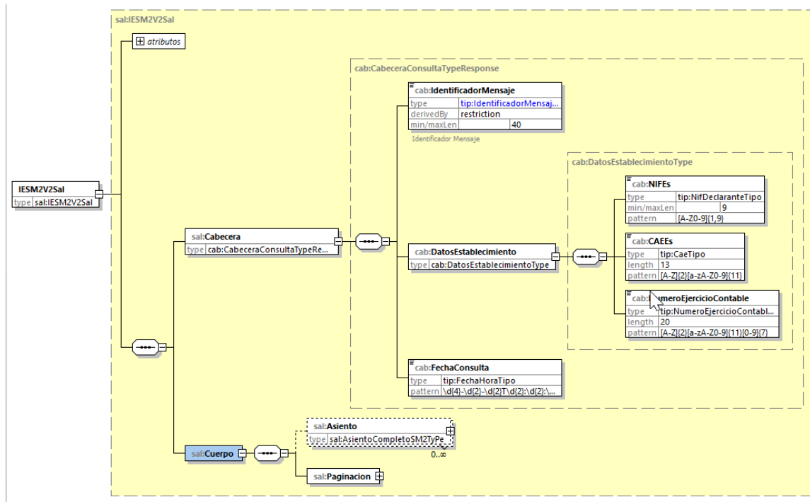
Figura 11: Estructura Básica Mensaje Salida
