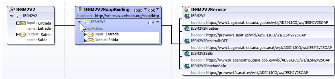
Figura 3: Esquema elemento de entrada
