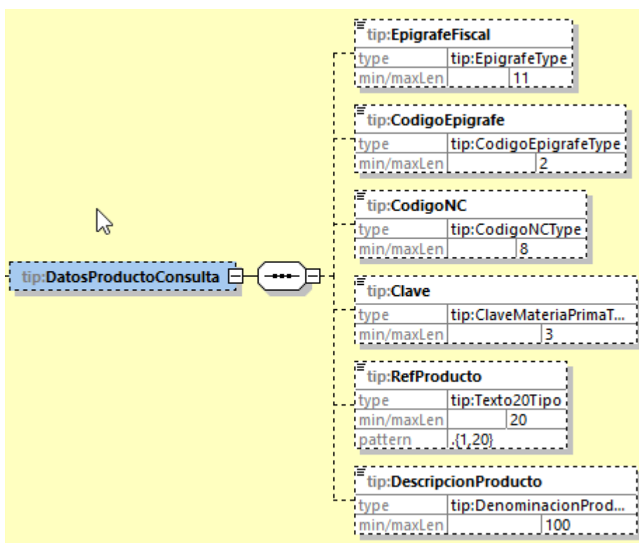
Figura 5: Datos Producto
