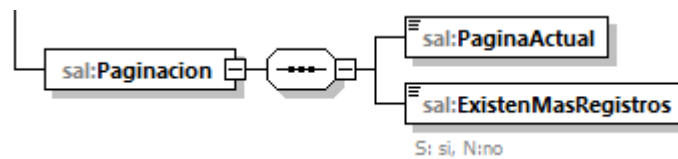
Figura 24: Paginación
